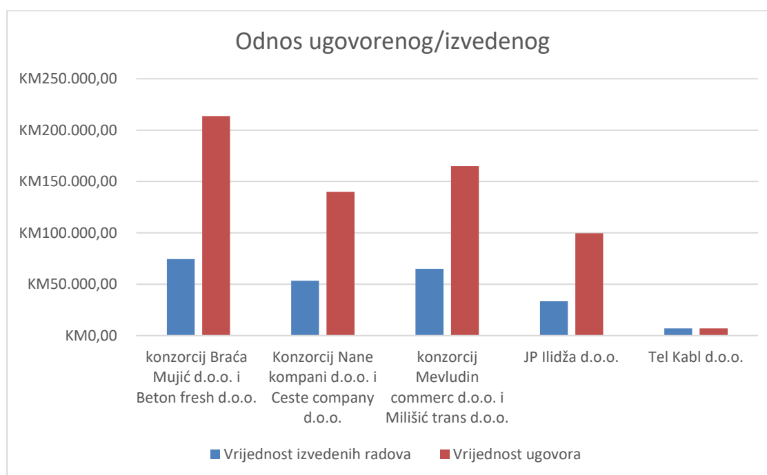
Slika 10.1. Rekapitulacija radova
